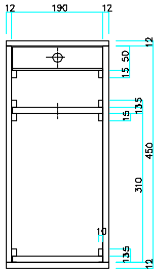
ケース本体
